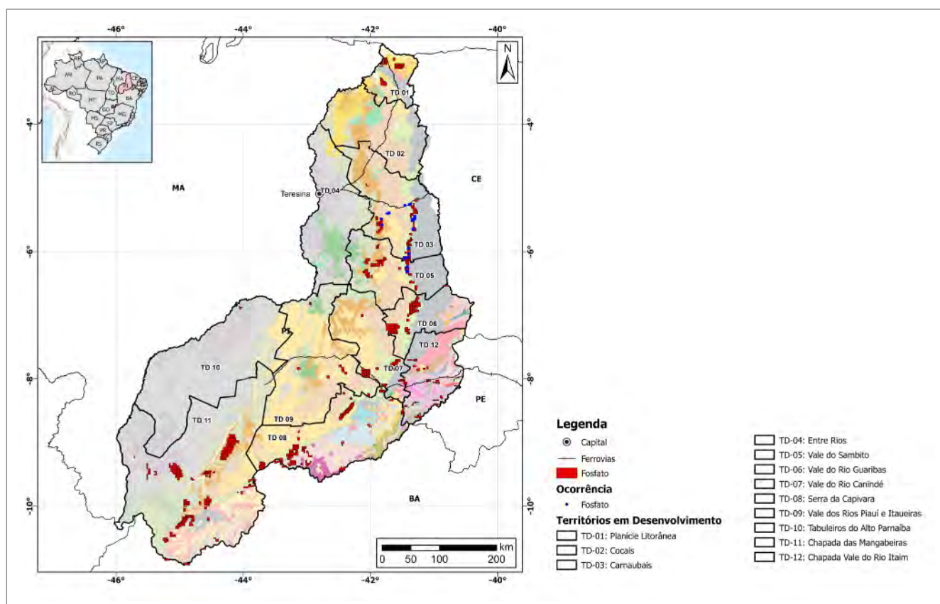
Figura 10.4 - Rocha fosfática no Piauí – Indicação de área com geologia favorável; Ocorrências e depósitos minerais e direitos minerários. Fonte: Moraes et al. 2015; figura reelaborada pela Plataforma P3M, 2023.
