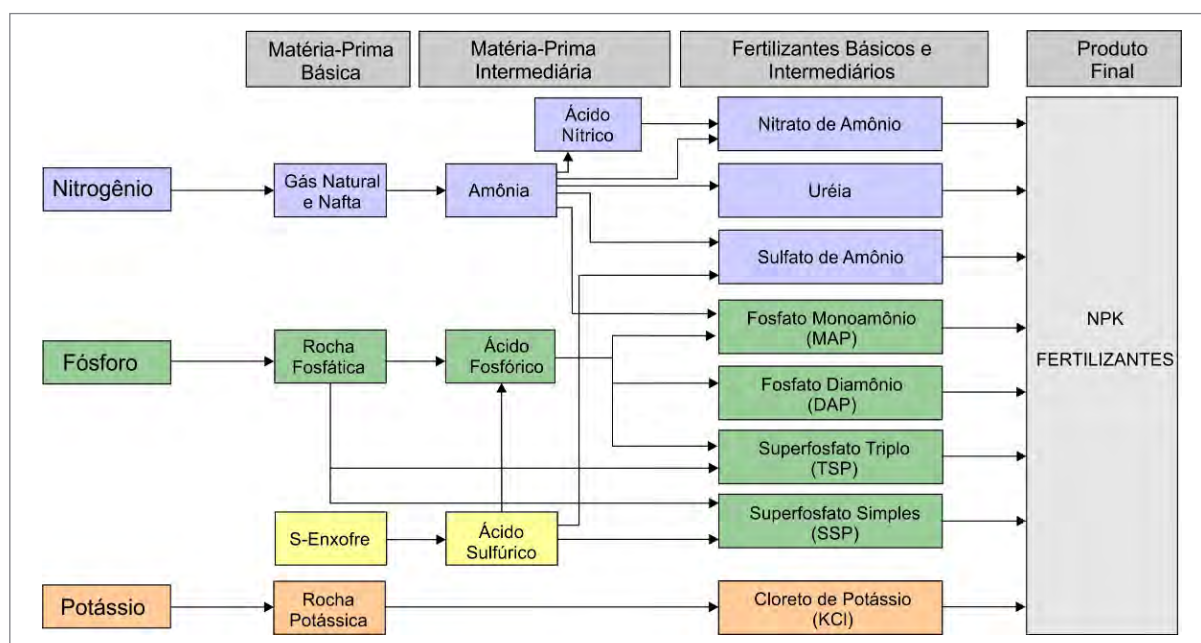
Figura 9.2 - Rocha fosfática e indústria de fertilizantes - Cadeia de produção. Fonte: Adaptado de Lobo, V. – UFRJ, 2006.
