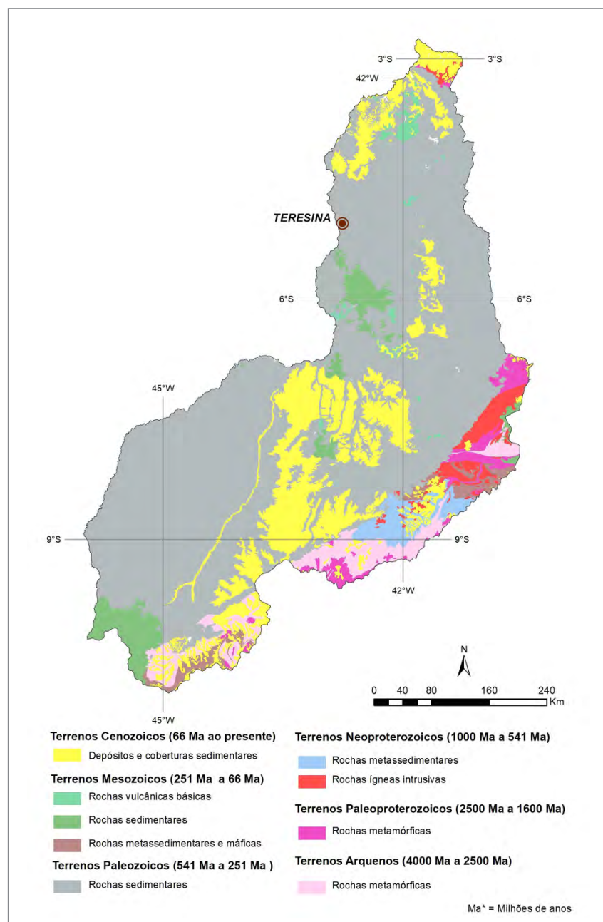
Figura 2.1 - Mapa geológico simplificado do estado do Piauí, contendo a distribuição das principais rochas e eras geológicas. Fonte: Modificado de Correia Filho et al. , 2006.
